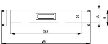
Рисунок 4 – Полка выдвижная серверная / Figure 4 – Sliding server shelf
